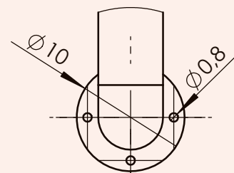
DETALLE A
