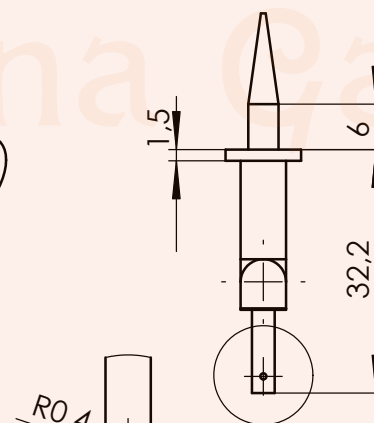
DETALLE B
